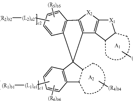
Formula 1E
