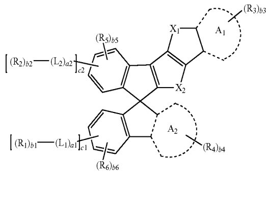
Formula 1E
